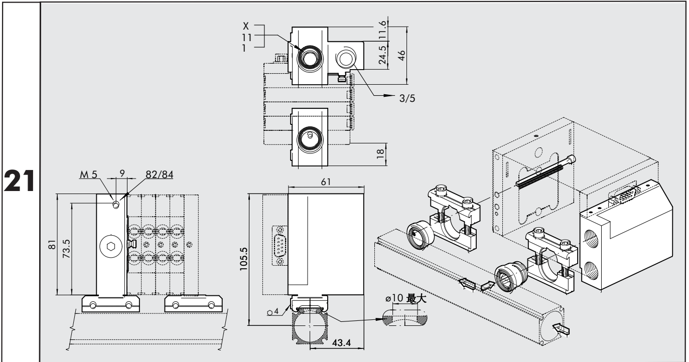
代号 说明 0227300203 PNEUMO-BUS 气动总线端板组件 备注: 订购带该端板的Multimach组合元件时, 请注明识别号21:M51-21...
