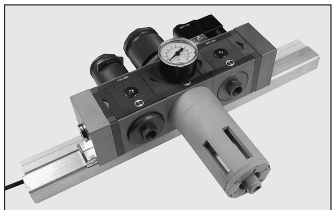
SKILLAIR 200 气源处理单元
