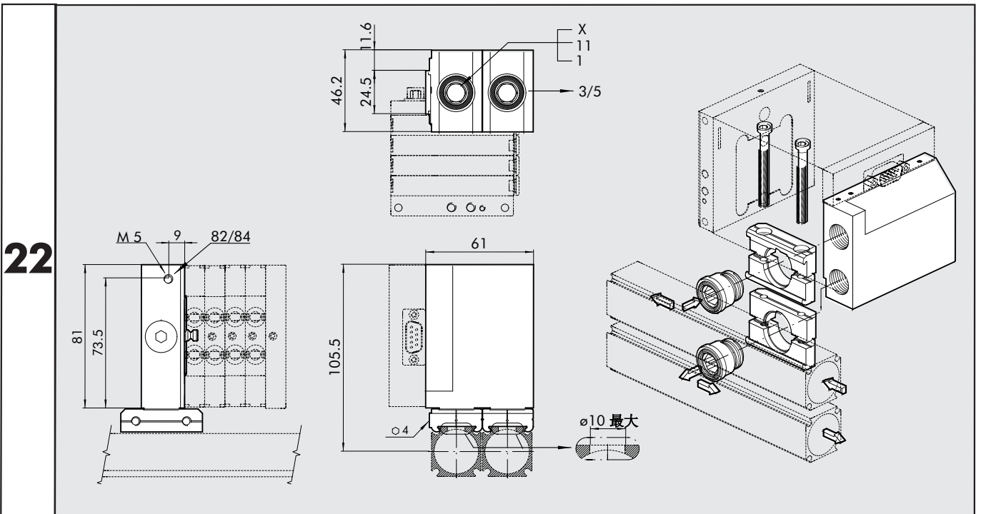
代号 说明 0227300204 PNEUMO-BUS 气动总线端板组件 + 输送排气口 备注: 订购带该端板的Multimach组合元件时, 请注明识别号22:M51-22...
