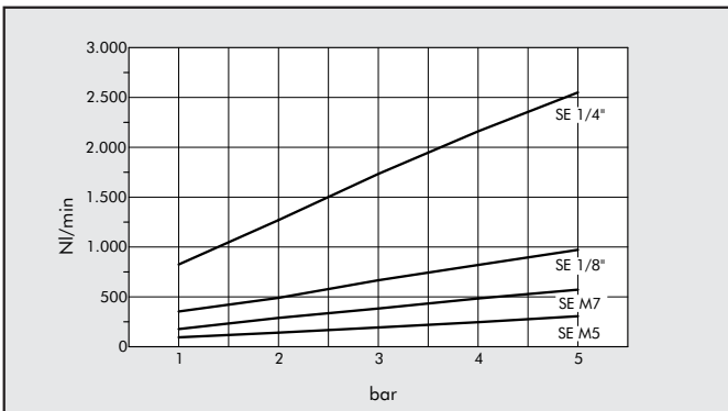
消声器，型号MW STT
