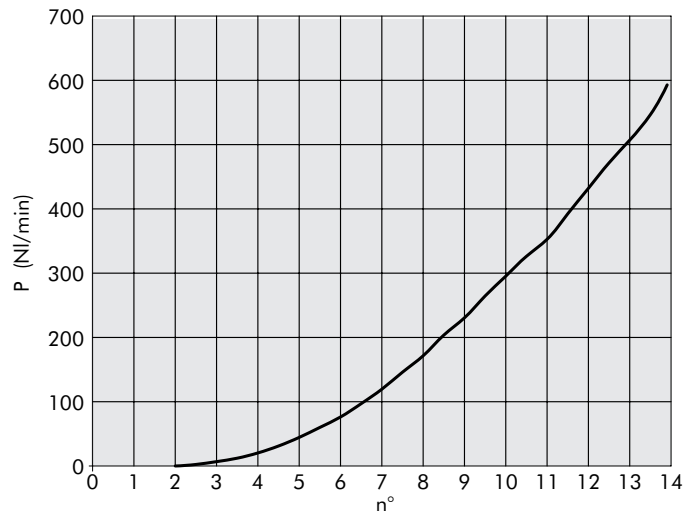
Ø10 管径的流量
