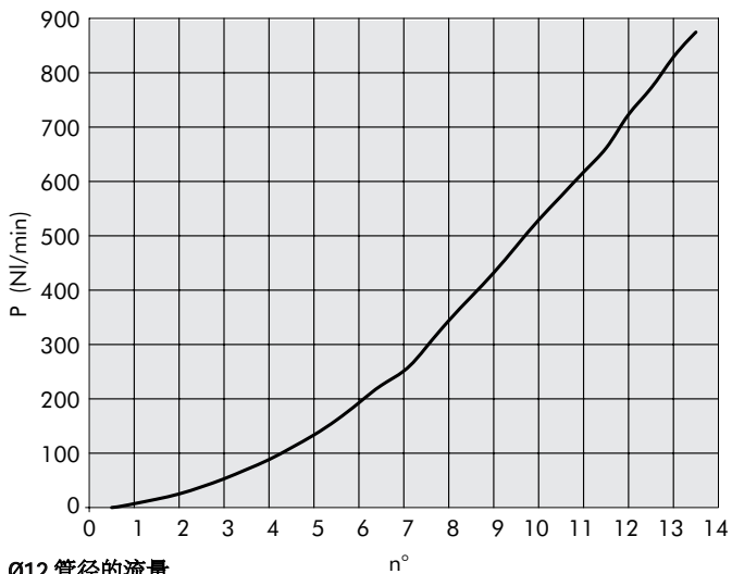
Ø12 管径的流量
