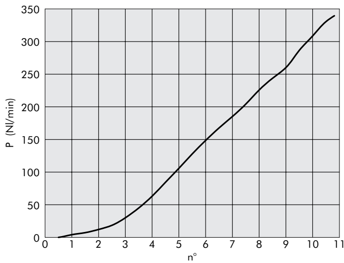
Ø6管径的流量
