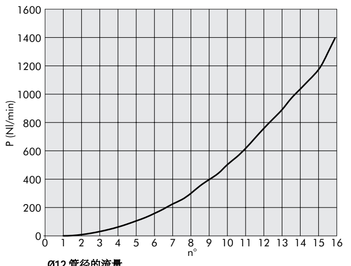
Ø12 管径的流量
