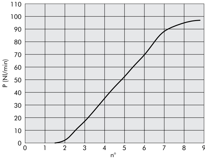
Ø6 管径的流量
