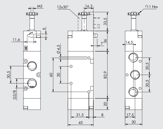
单稳型 5/2 3/8" 手杆操作
