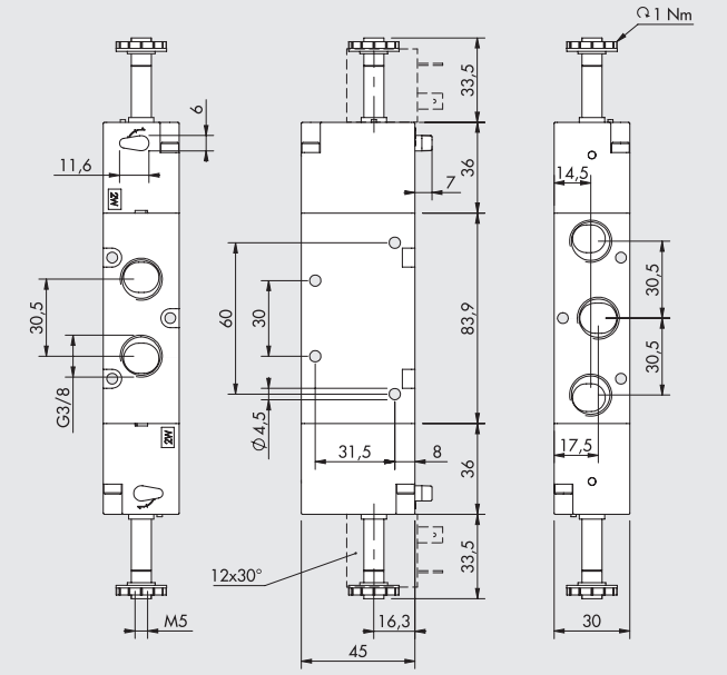
双稳型 5/2 3/8" 手杆操作
